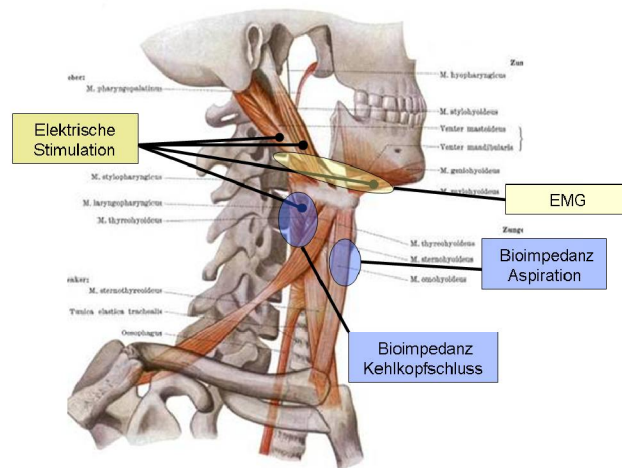
Abbildung 1: Modell des geplanten Mess- und Stimulationsystems als Grundlage für eine geregelte Schluckneuroprothese. Gekennzeichnet sind die Stimulationsorte und die Messpunkte für EMG und Bioimpedanz.
